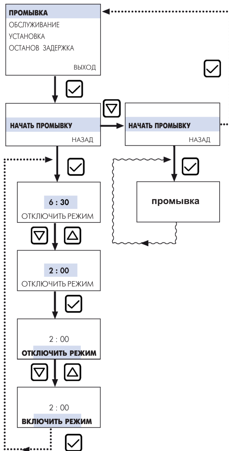
Рис. 19: Программируемая процедура "ПРОМЫВКА"
