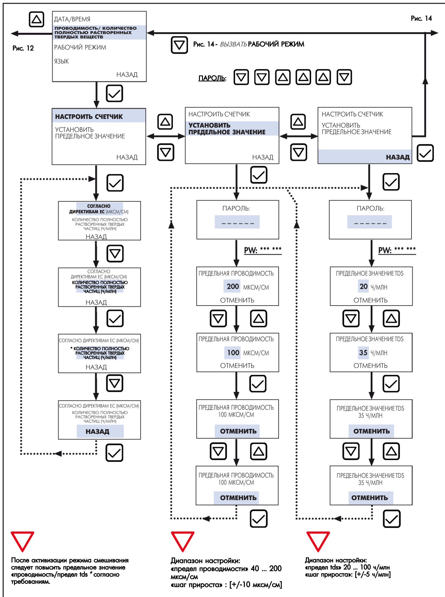
Рис. 13. Процесс программирования: ПРОВОДИМОСТЬ / Значение электропроводимости/общего количества растворенных твердых веществ
