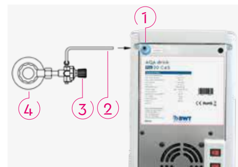
Рис. 11: Подключение баллона со сжатым CO 2
