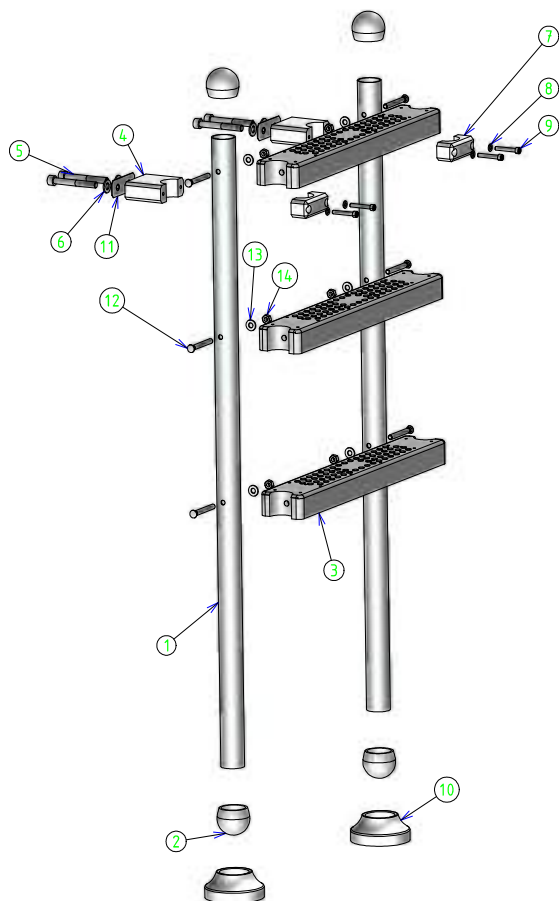
Рисунок 29 – Монтаж лестницы
