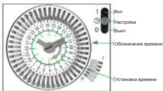
Рисунок 58 – Лицевая поверхность таймера системы фильтрации
