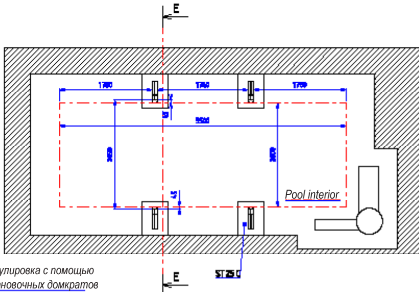
Рисунок 3 – а в b - Установка домкратов на опорные стойки
