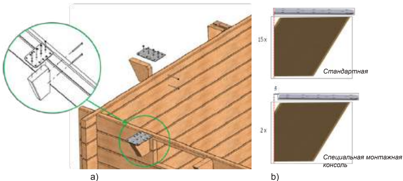
Рисунок 14 – а и б – Монтаж металлических пластин на консолях бортиков
