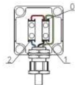
Рисунок 57 – Блок ключевого управления
