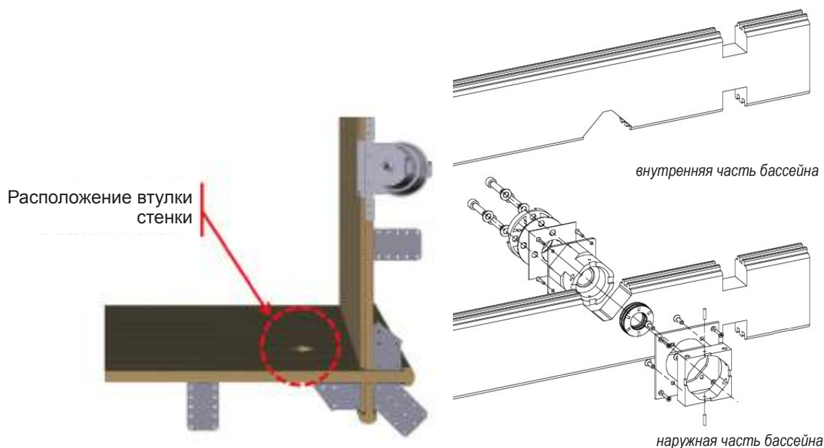
Рисунок 26 – Расположение втулки стенки
