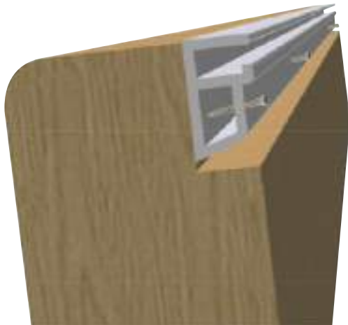
Рисунок 30 – Установка рейки
