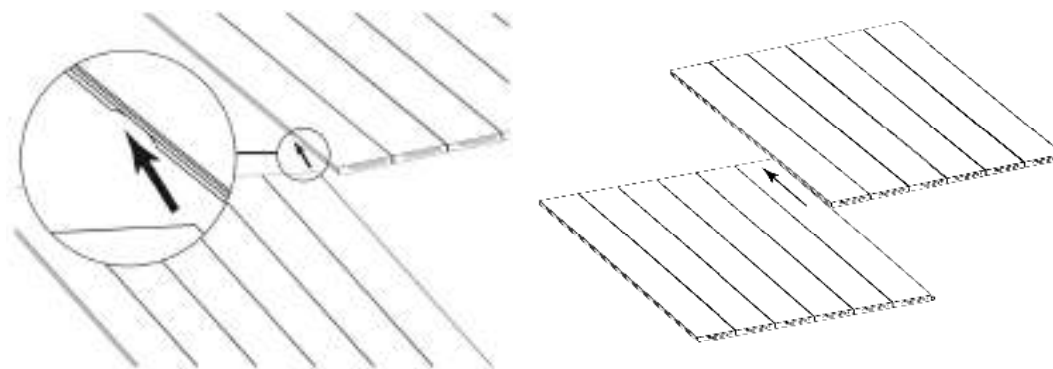
Рисунок 44 – Сборка полотна
