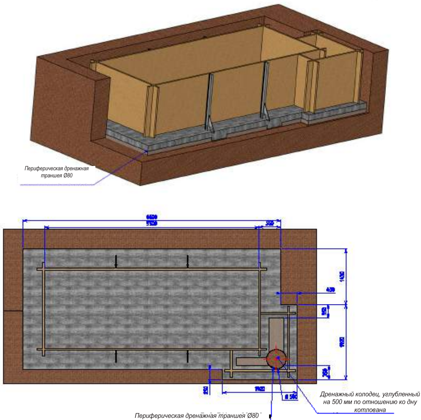
Рисунок 1 – Схема дренажной системы
