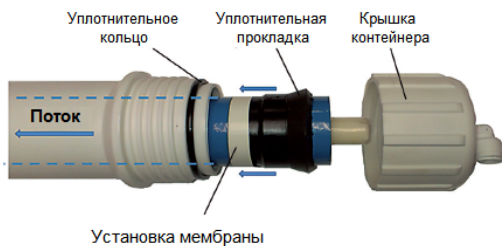
Установка мембраны
